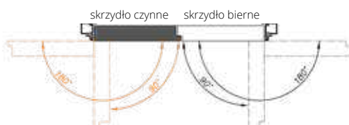
C. Drzwi lewe otwierane na zewnątrz
