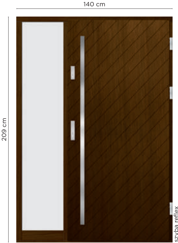
NS 41 Widok od zewnątrz Dostawka stała w ościeżnicy
