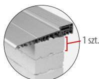
wkładka termoizolacyjna wys. 30 mm x szer. 64 mm - za dopłatą 50 zł
