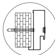
otwór montażowy w otworze w centrum profilu na pierś ościeżnicy
