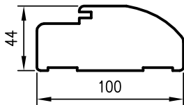
Profil OP SOFT
